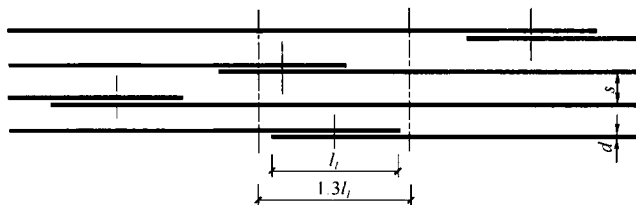
图 1 钢筋绑扎搭接接头连接区段及接头面积百分率
